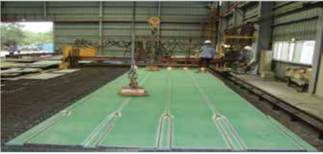
STEP 3 : 가조립
