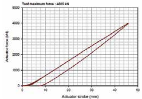
〈유압가력기의 하중-변위 그래프〉
