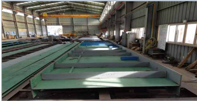
· STEP 4 : 공장 가조립
