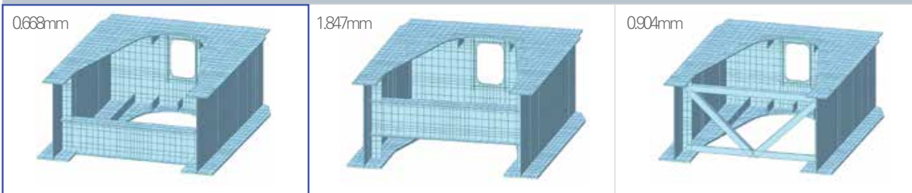
가로보 위치검토
