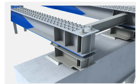
거더 단부
